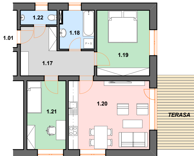
PŮDORYS BYTU
